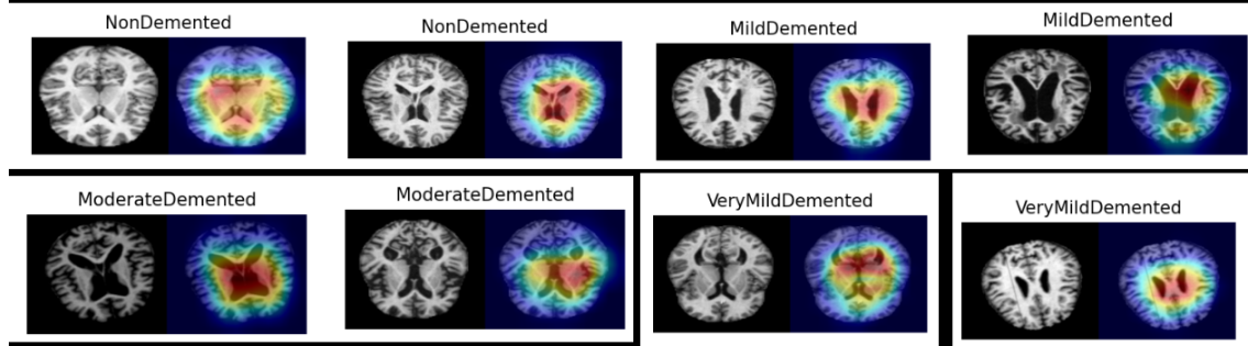
Figura B.3: Esempi di mappe di attivazione (Grad-CAM) ottenute dal modello Custom-CNN per le quattro classi considerate: NonDemented , MildDemented , ModerateDemented e VeryMildDemented . Per ciascun esempio sono mostrate l'immagine MRI originale (a sinistra) e la corrispondente heatmap sovrapposta (a destra), che evidenzia le regioni cerebrali maggiormente rilevanti per la decisione del modello. Le aree in rosso indicano le zone con maggiore contributo alla classificazione.
