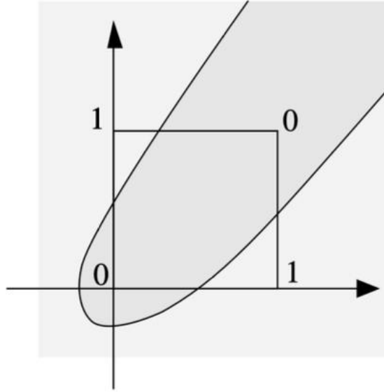
Figura 2.4: Schema del problema XOR: i vertici (0,1) e (1,0) appartengono alla classe 1, (0,0) e (1,1) alla classe 0. Nessuna frontiera lineare può separare le classi; è necessaria una frontiera non lineare (ottenibile con uno strato nascosto).
